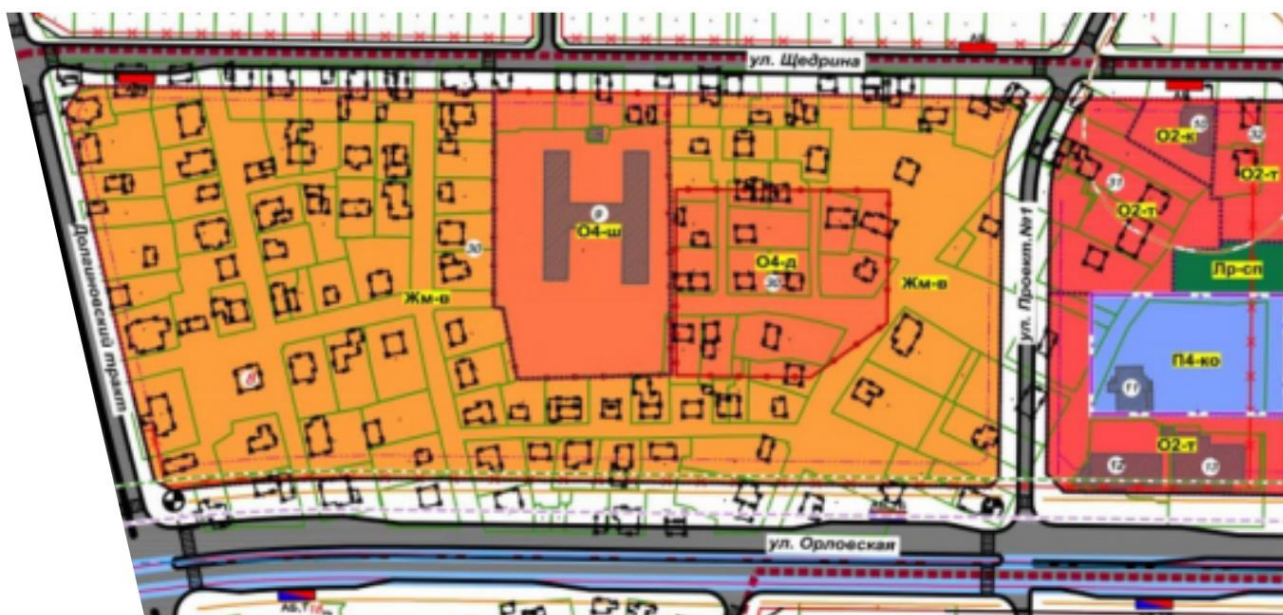
Фрагмент градостроительного проекта детального планирования на указанную территорию.
